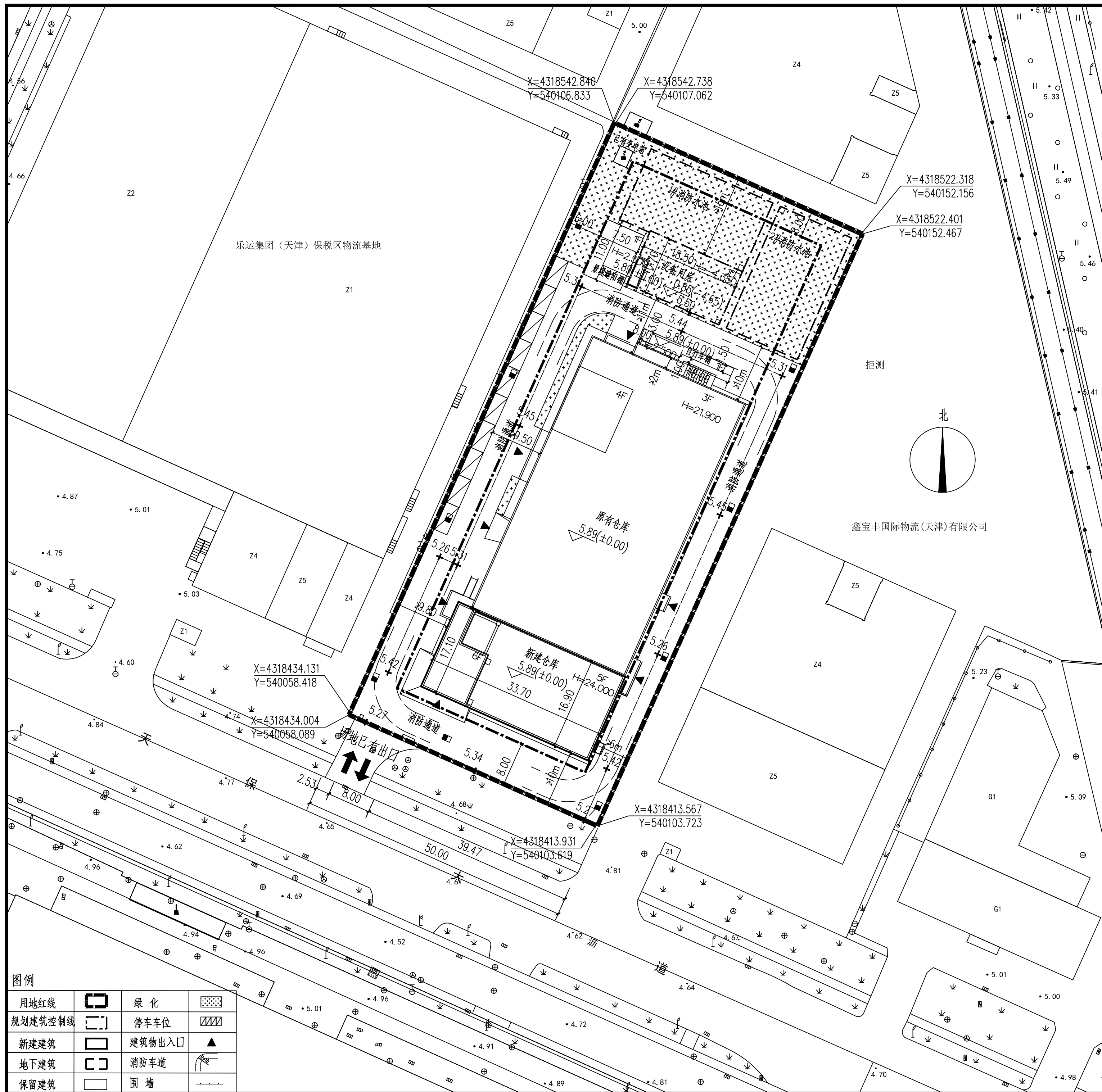
总平面图 1:500
